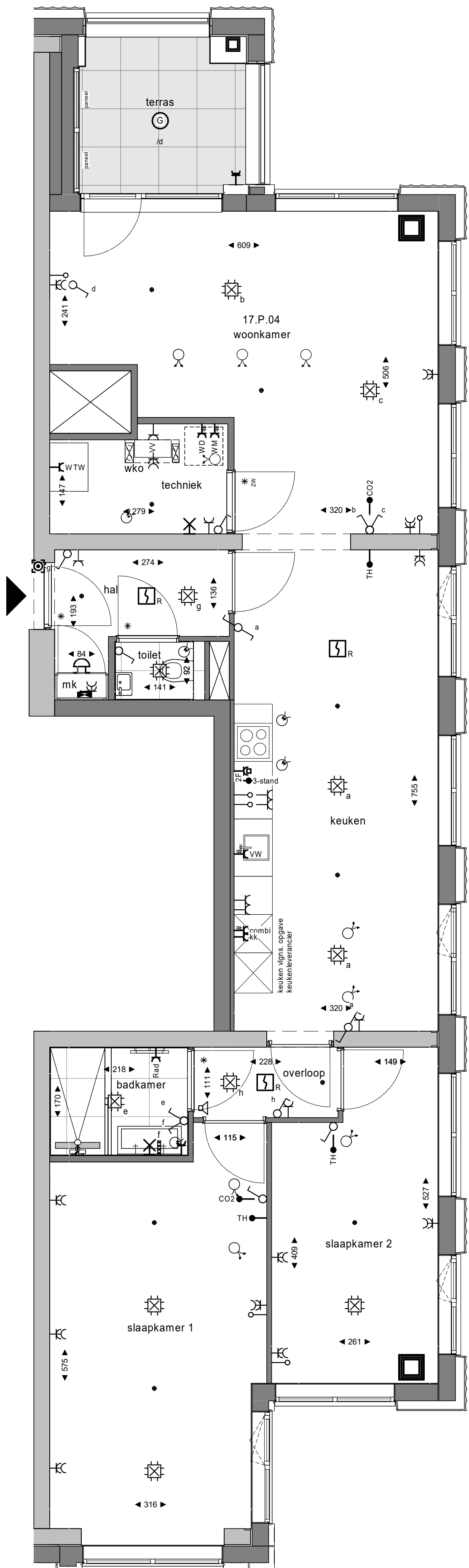
plattegrond 1 : 50 17e verdieping
